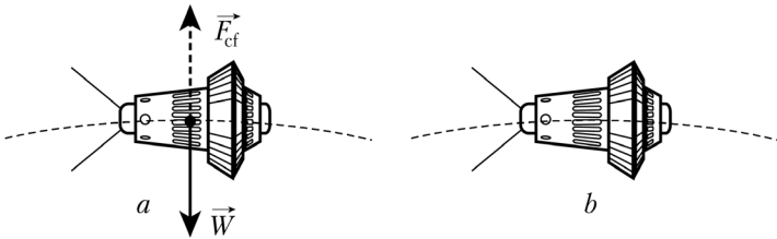
Рис. 1.2. Силы, действующие на космический корабль на орбите в ньютоновской инерциальной системе отсчета (а) и системе отсчета, выделенной в ОТО (б). Здесь W — сила тяжести, а F_{cf} — центробежная сила
